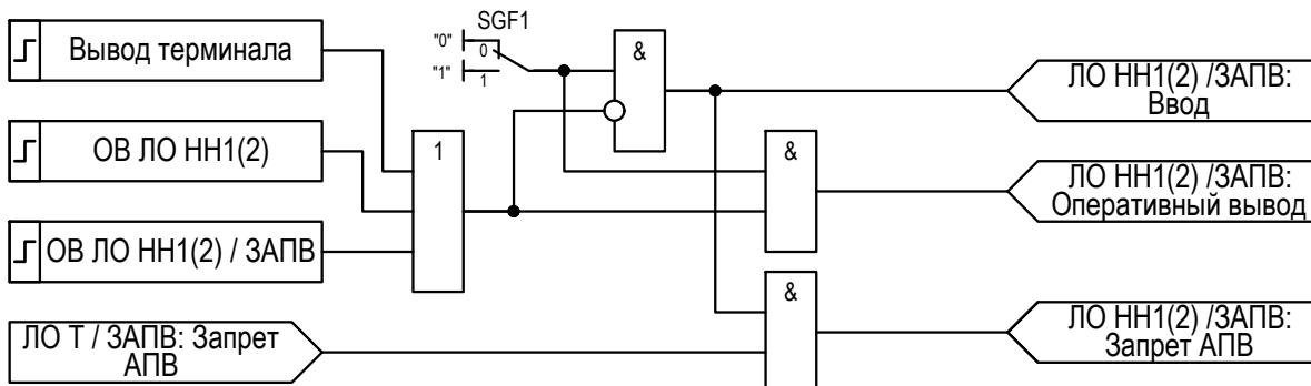
Рисунок 2.31 – Функциональная схема «Запрет АПВ»
